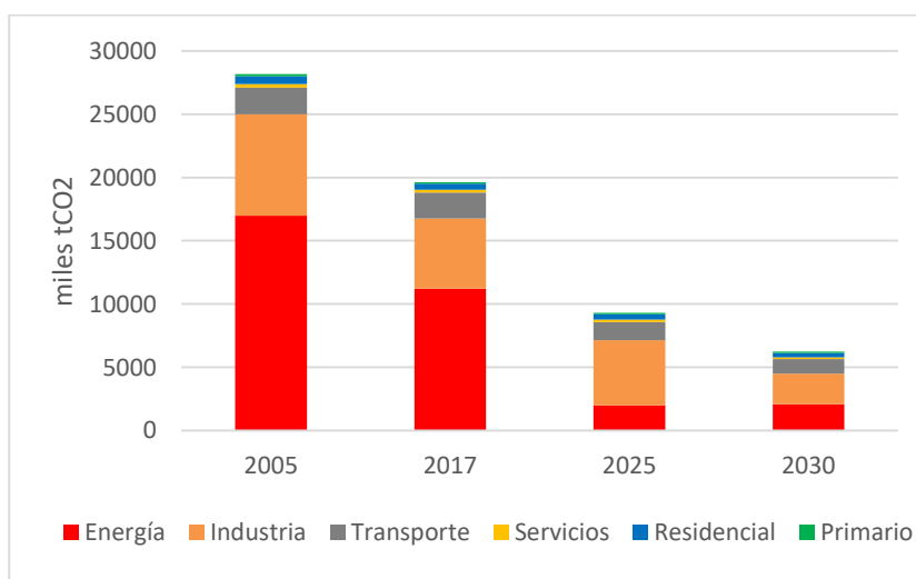
Figura 64: Evolución del reparto de emisiones de CO 2eq procedentes del procesamiento de energía en Asturias según escenario objetivo. Fuente: FAEN
