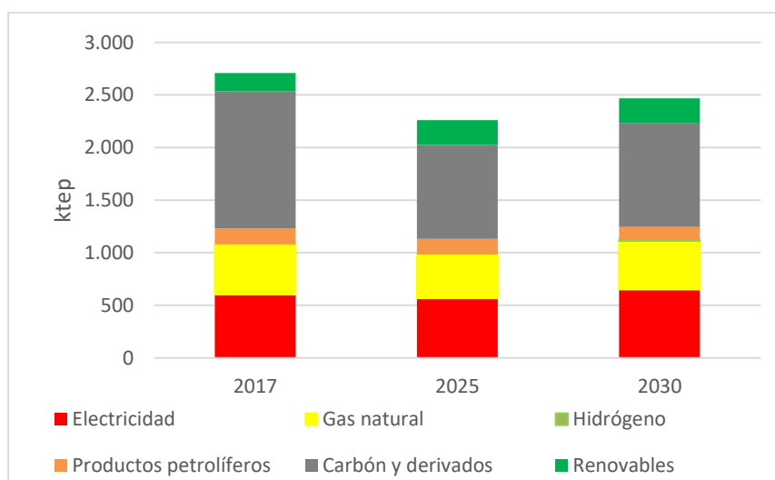
Figura 31. Evolución del consumo de energía final en la industria por fuentes según escenario tendencia Fuente: FAEN
