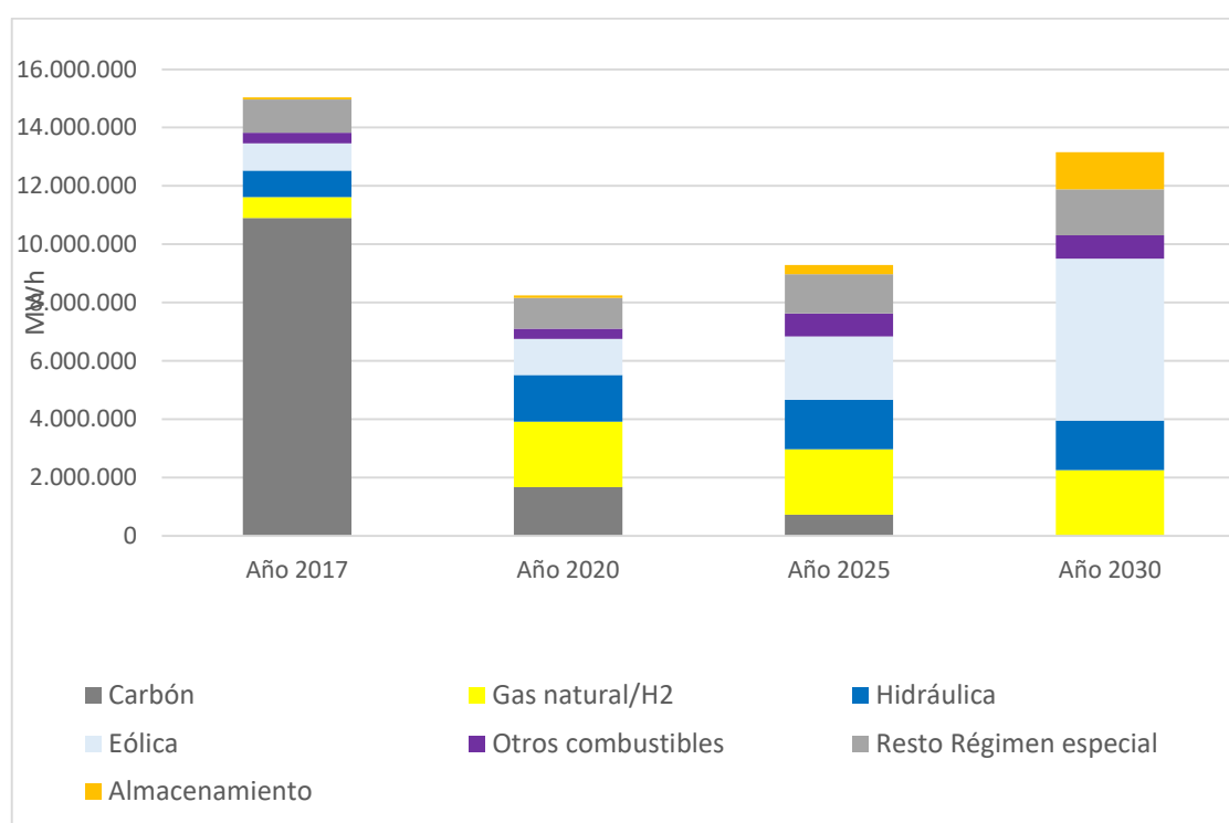
Figura 16. Evolución de la generación de electricidad en el periodo 2017-2030 según escenario objetivo. Fuente: FAEN
